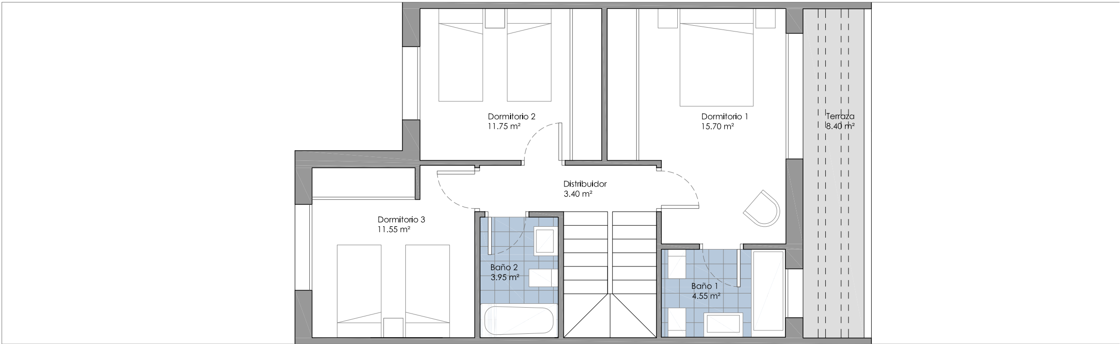
P. PRIMERA
